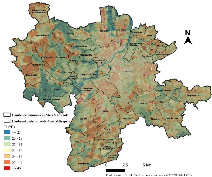
Figure 2 : Thermographie de surface Landsat de Metz Métropole (09/08/2020).
