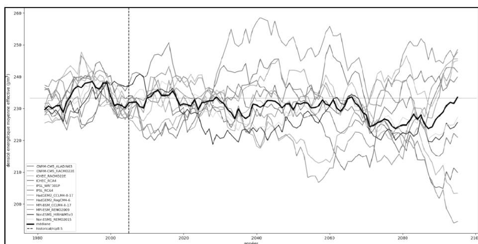
Figure 5 : Evolution de la densité énergétique moyenne en France au XXI e siècle sur l'ensemble de 12 simulations RCP8.5 du jeu DRIAS-2020
