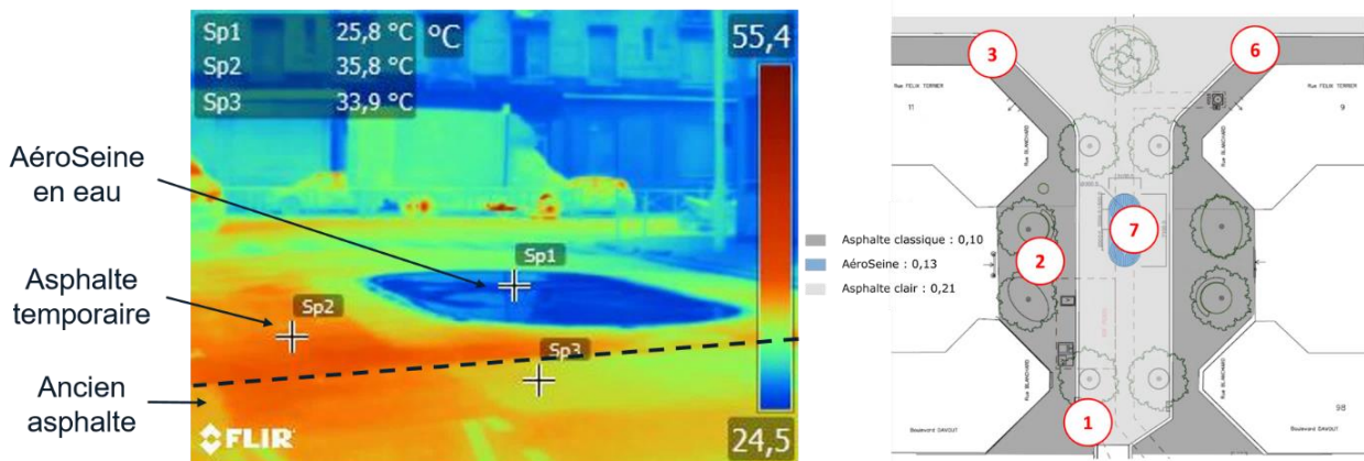
Figure 12 : Photographie infrarouge du dispositif en eau (gauche) et plan avec albédos correspondants (droite)
