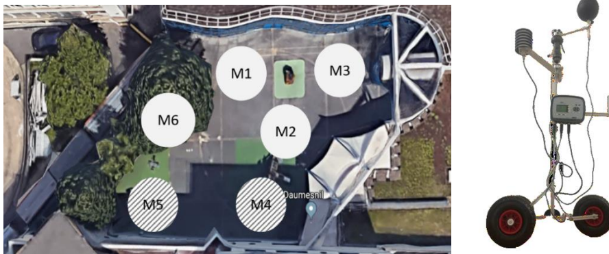
Figure 39 : Points de mesures dans la cour (gauche) et photo de la station mobile (droite).
