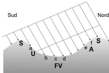
Fig. 1 : Les différents topo-climats associés à la montagne. Nous donnons ici comme exemple les noms locaux des Alpes françaises. A-B : versant sud (Adret), E-F : versant nord (Ubac), C-D : Fond de vallée et S : Sommet ou Ligne de crête..
