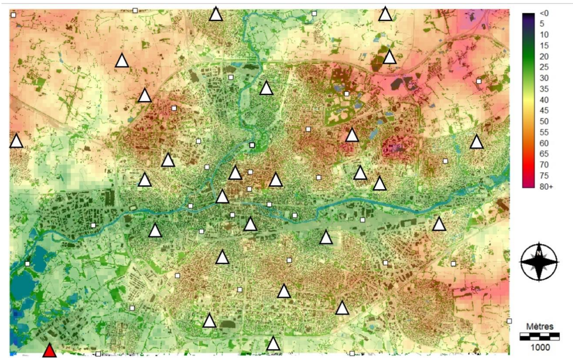
Figure 1. Réseau d'observation climatologique sur Rennes en 2020 : triangles blancs = stations automatiques Davis ; triangle rouge = station synoptique Météo France de Saint Jacques de la Lande ; petits carrés blancs = micro-capteurs HOBO ; Modèle numérique de terrain (couleur) et bâti (noir) en arrière-plan.
